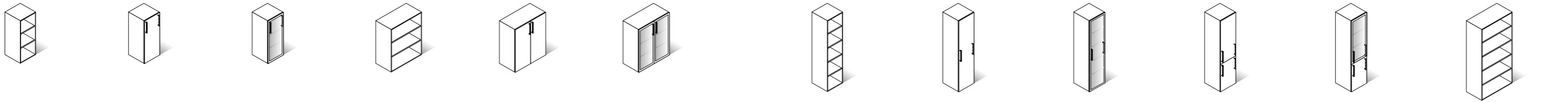
Libreria media a giorno Medium height open cabinet OLM45G cm. 45x47x118 h. Libreria media con ante in legno dx/sx Medium height cabinet with wooden door (r/l) OLM45LD cm. 45x47x118 h. OLM45LS cm. 45x47x118 h. Libreria media con ante in vetro temperato dx/sx Medium height cabinet with toughened glass door (r/l) OLM45VTD cm. 45x47x118 h. OLM45VTS cm. 45x47x118 h. Libreria media a giorno Medium height open cabinet OLM90G cm. 90x47x118 h. Libreria media con ante in legno Medium height cabinet with wooden doors OLM90L cm. 90x47x118 h. Libreria media con ante in vetro temperato Medium height cabinet with toughened glass doors OLM90VT cm. 90x47x118 h. Libreria alta a giorno Tall open cabinet OLA45G cm. 45x47x195 h. Libreria alta con ante in legno dx/sx Tall cabinet with wooden door (r/l) OLA45LD cm. 45x47x195 h. OLA45LS cm. 45x47x195 h. Libreria alta con ante in vetro temperato dx/sx Tall cabinet with toughened glass door (r/l) OLA45VTD cm. 45x47x195 h. OLA45VTS cm. 45x47x195 h. Libreria alta con ante in legno dx/sx Tall cabinet with wooden doors (r/l) OLA45LLD cm. 45x47x195 h. OLA45LLS cm. 45x47x195 h. Libreria alta con ante in legno e in vetro temperato dx/sx Tall cabinet with wooden door and toughened glass door (r/l) OLA45LVTD cm. 45x47x195 h. OLA45LVTS cm. 45x47x195 h. Libreria alta a giorno Tall open cabinet OLA90G cm. 90x47x195 h.
