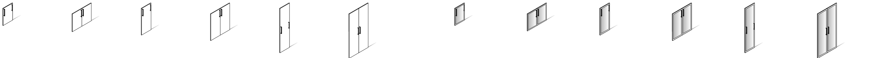
Anta bassa per librerie in legno dx/sx Low door for wooden cabinet (right/left) OLABD1 cm. 44,7x1,9x76,2 h. OLABS1 cm. 44,7x1,9x76,2 h. Coppia di ante basse per librerie in legno Low doors for wooden cabinet OLAB2 cm. 89,4x1,9x76,2 h. Anta media per librerie in legno dx/sx Medium height door for wooden cabinet (right/left) OLAMD1 cm. 44,7x1,9x114,6 h. OLAMS1 cm. 44,7x1,9x114,6 h. Coppia di ante medie per librerie in legno Medium height doors for wooden cabinet OLAM2 cm. 89,4x1,9x114,6 h. Anta alta per librerie in legno dx/sx Tall door for wooden cabinet (right/left) OLAAD1 cm. 44,7x1,9x191,4 h. OLAAS1 cm. 44,7x1,9x191,4 h. Coppia di ante alte per librerie in legno Tall doors for wooden cabinet OLAA2 cm. 89,4x1,9x191,4 h. Anta bassa in vetro temperato per librerie in legno dx/sx Low toughened glass door for wooden cabinet (right/left) OLABDV1 cm. 44,7x1,9x76,2 h. OLABSV1 cm. 44,7x1,9x76,2 h. Coppia di ante basse in vetro temperato per librerie in legno Low toughened glass doors for wooden cabinet OLABV2 cm. 89,4x1,9x76,2 h. Anta media in vetro temperato per librerie in legno dx/sx Medium height toughened glass door for wooden cabinet (right/left) OLAMDV1 cm. 44,7x1,9x114,6 h. OLAMSV1 cm. 44,7x1,9x114,6 h. Coppia di ante medie in vetro temperato per librerie in legno Medium height toughened glass doors for wooden cabinet OLAMV2 cm. 89,4x1,9x114,6 h. Anta alta in vetro dx/sx temperato per librerie in legno Tall toughened glass door for wooden cabinet (right/left) OLAADV1 cm. 44,7x1,9x191,4 h. OLAASV1 cm. 44,7x1,9x191,4 h. Coppia di ante alte in vetro temperato per librerie in legno Tall toughened glass doors for wooden cabinet OLAAV2 cm. 89,4x1,9x191,4 h.
